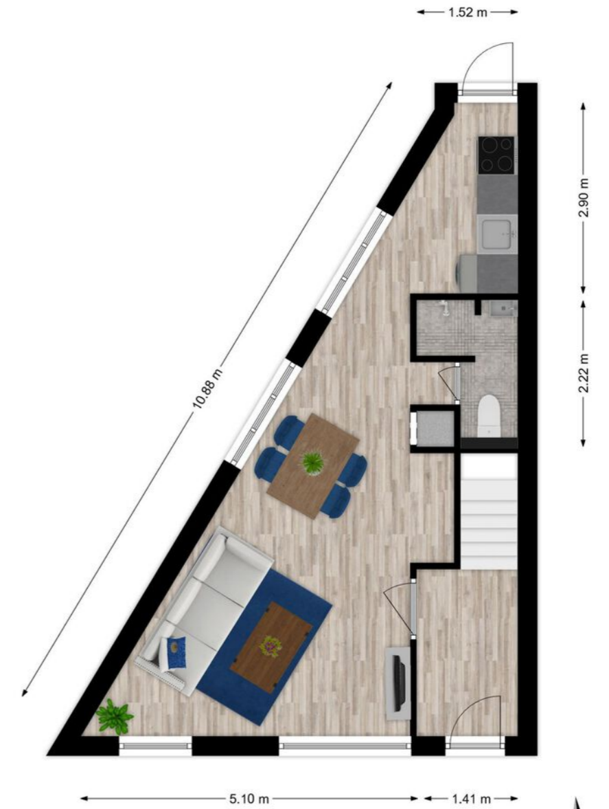
Begane grond, Rhijnvis Feithstraat 14-BS te Utrecht Deze plattegronden zijn opgemaakt voor indicatieve doeleinden. Hieraan kunnen geen rechten worden ontleend.
